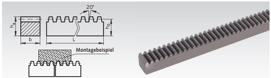
Die Zahnstangen werden mit Überkopfräser verzahnt. Dadurch entstehen Minus-Toleranzen. Maß h_a und h_0 bis Modul 2 -0,2 mm, Modul 2,5-4 -0,3 mm, Modul 5-8 -0,4 mm
