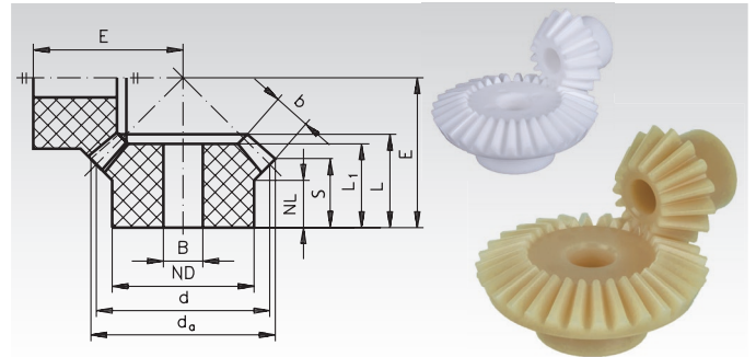
Zeichnung zeigt Übersetzung 1:1, Foto zeigt Übersetzung 2:1
