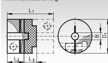
Klemmnabenausführung
