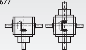
Ausführung 30 Ausführung 60
