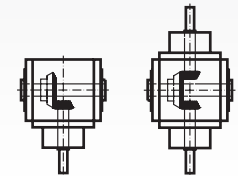
Ausführung 70 Ausführung 80
