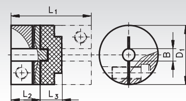
Klemmnabenausführung
