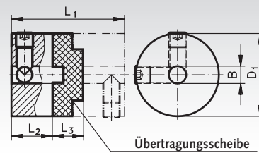
Stellschraubenausführung
