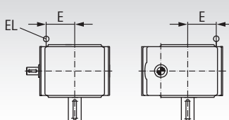
Montážna pozícia 5
